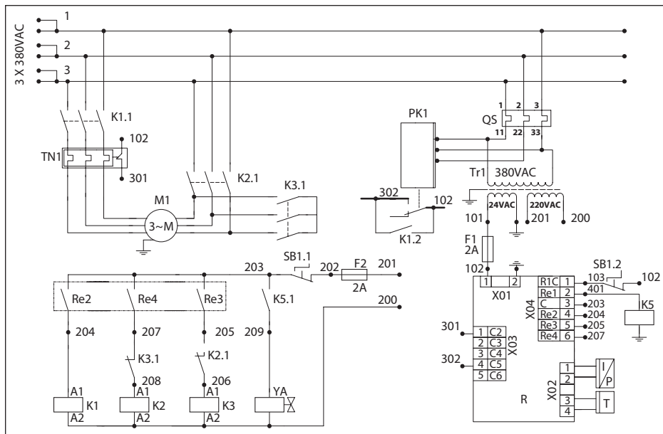
Рис. 2.6.2. Схема электрическая А11.. – А22.., АR11.. – АR22.., АRD11.. – АRD22.*
