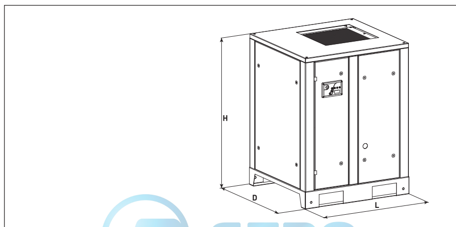
Рис. 3.2.1. Размеры компрессора А07.. – А22.
