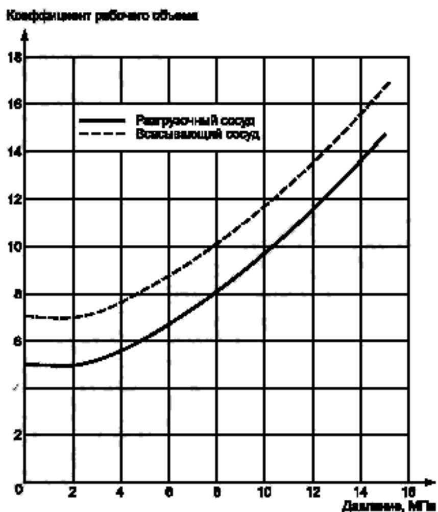
Рисунок В.1 — Объем буферных емкостей
