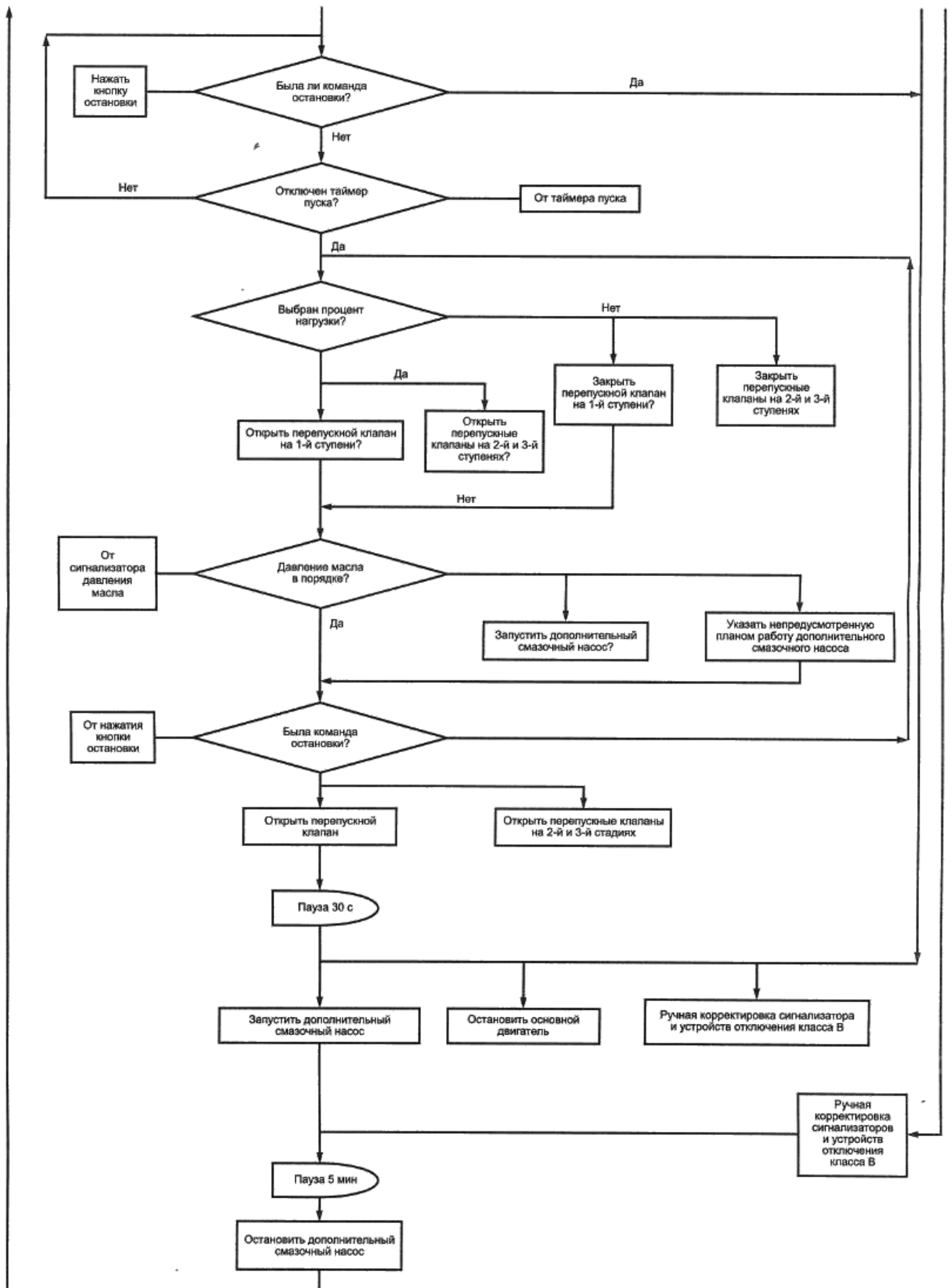
Рисунок С.1, лист 2
