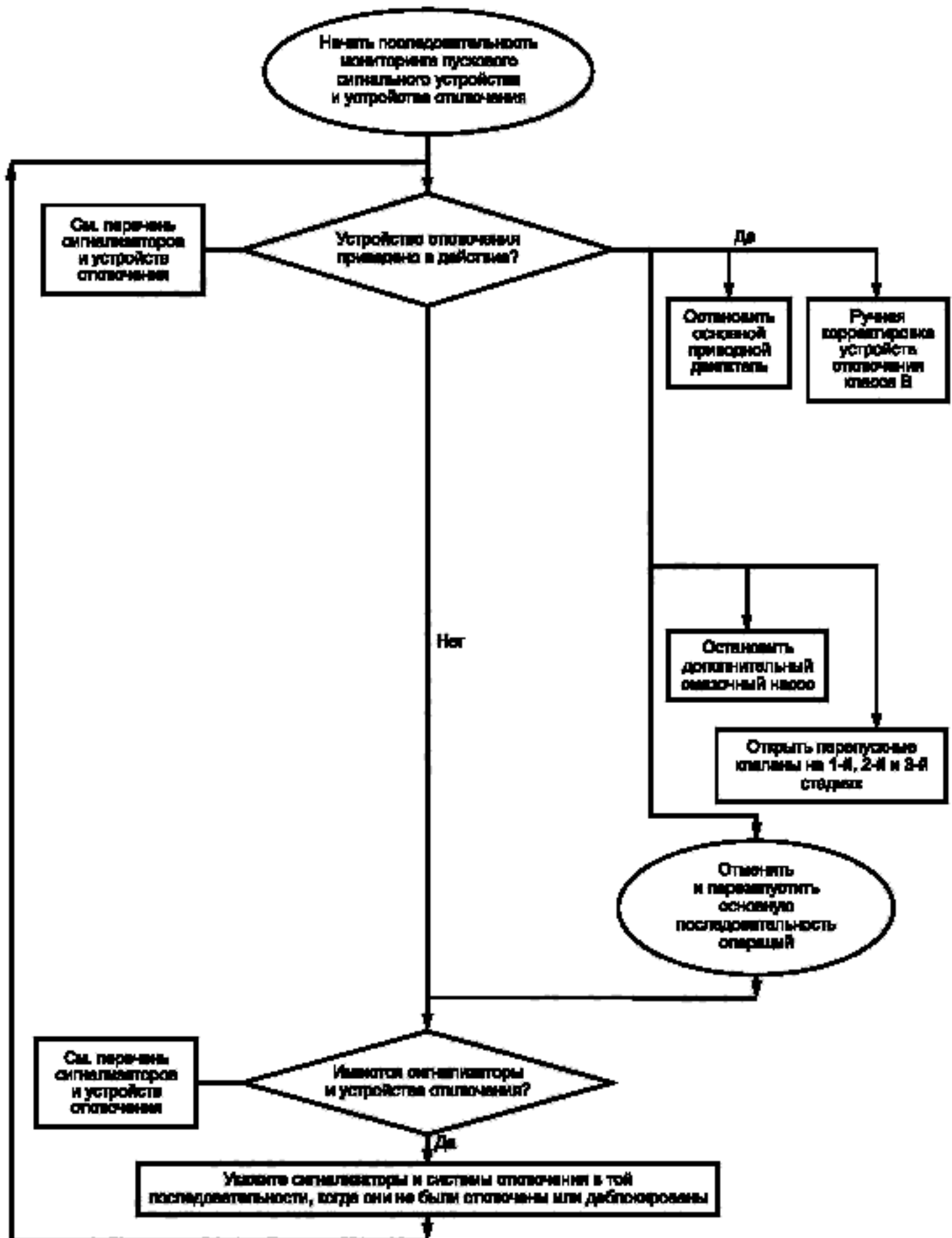
Рисунок С.2 — Типовая схема отключения
