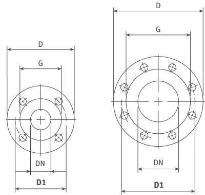
ФЛАНЦЫ НАСОСА
