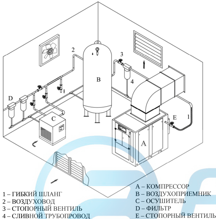
Рисунок 2.1 : УСТАНОВКА
