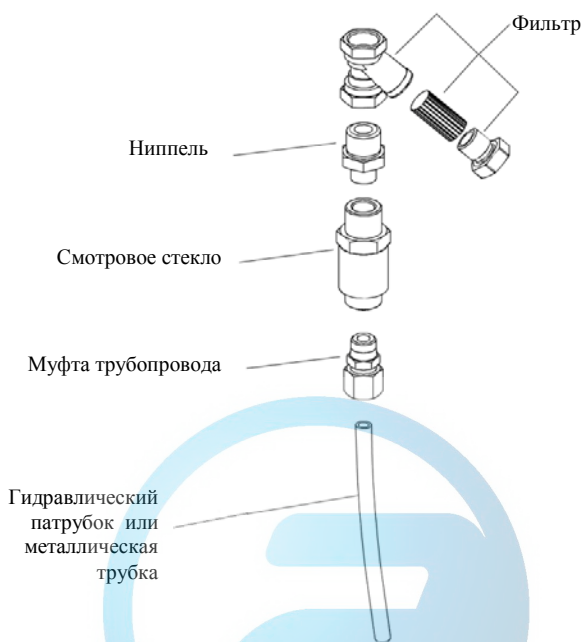
Рисунок 5.5 : СБОРКА СИСТЕМЫ ОТКАЧКИ
