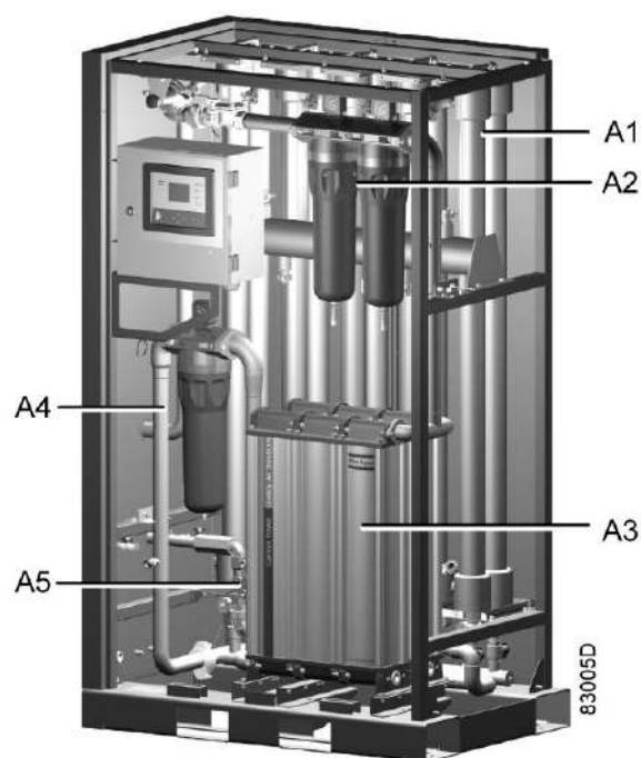
Вид NGM 4 - NGM 7
