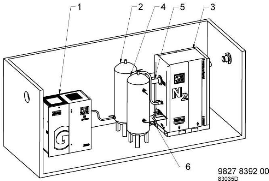
Предложение по установке для NGM (стандартная установка с компрессором GA)
