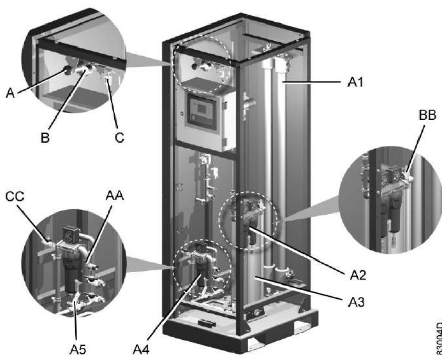
Вид с NGM 1 до NGM 3
