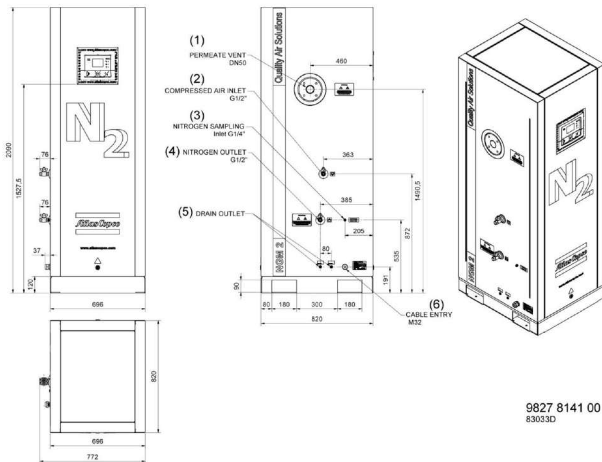
Размеры NGM 1 - NGM 3
