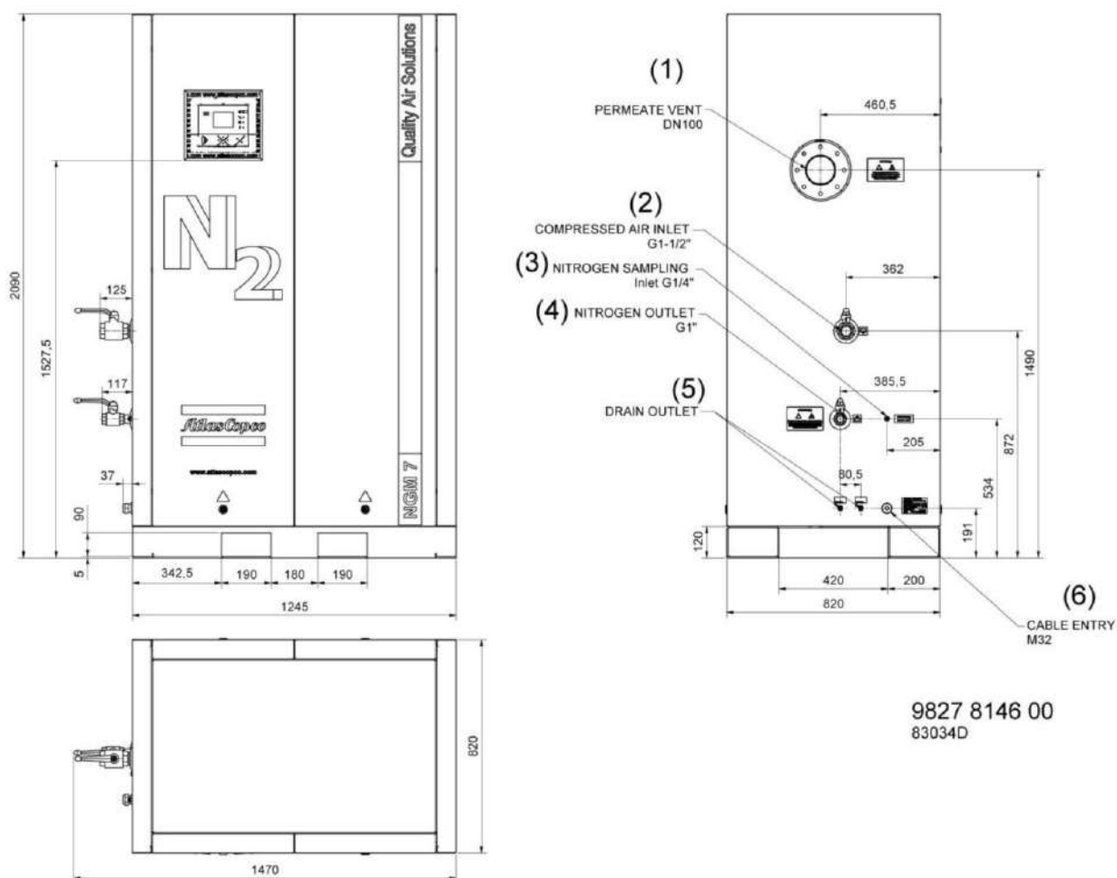
Размеры NGM 4 - NGM 7
