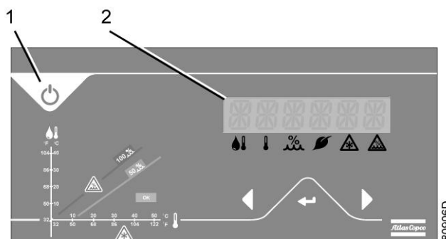
Панель управления
