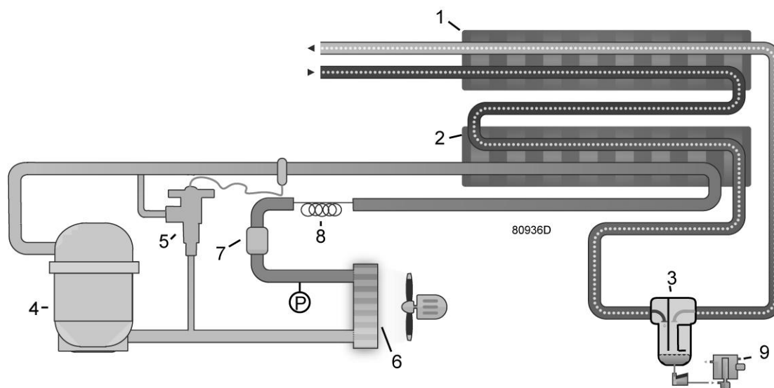
Схема потока
