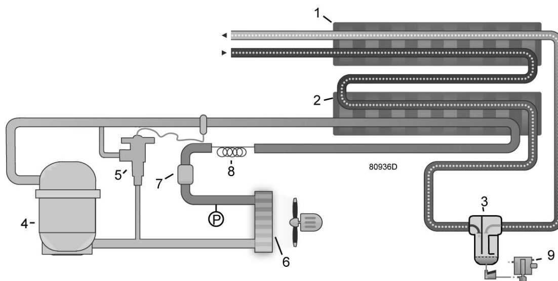
Схема потока
