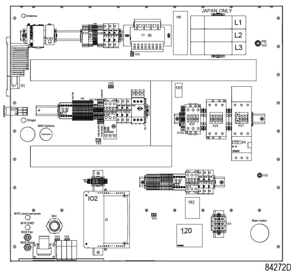
Установки с фиксированной скоростью - типовой вид
