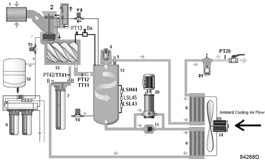
Компрессор с воздушным охлаждением
