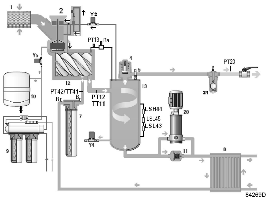
Компрессоры с водяным охлаждением
