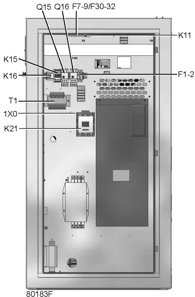
Установки с регулируемой скоростью - типовой вид
