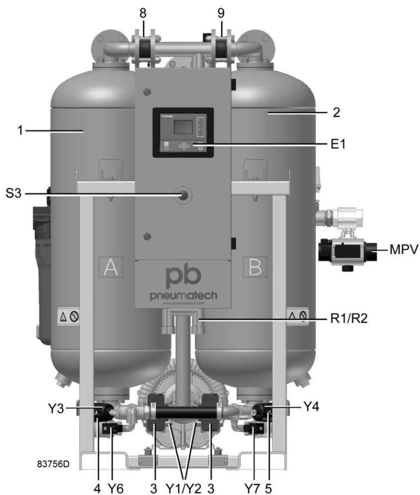
Вид спереди
