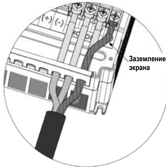
Рис. 8-3. Заземление экранированного кабеля
