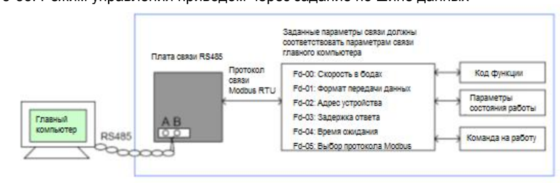
Рис. 5-33. Режим управления приводом через задание по шине данных
