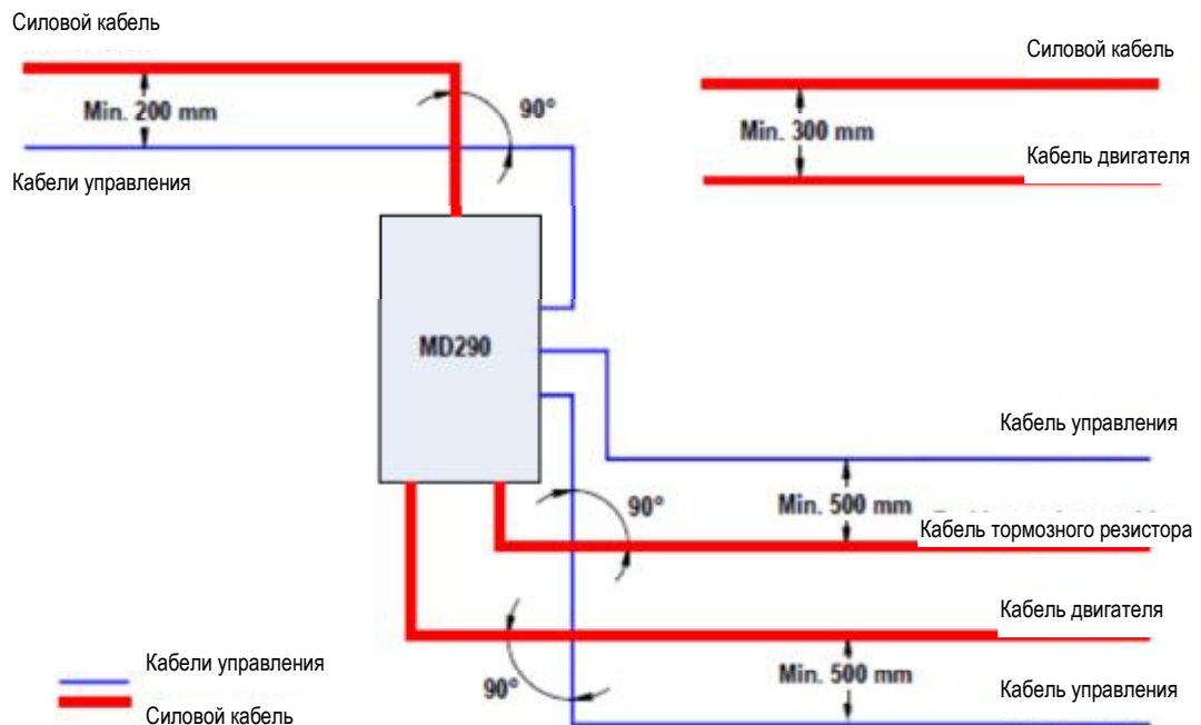
Рис. 8-4. Схема прокладки кабелей
