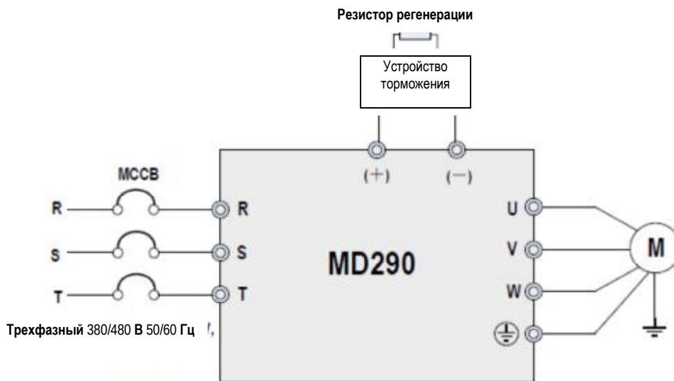
Рис. 4-3. Проводка главного контура MD290 (трехфазный ток 380 – 480 В, от 90G/110P до 110G/132P)
