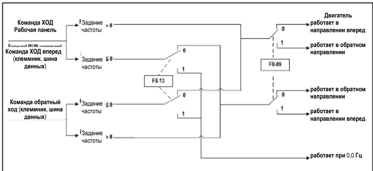
Рис. 5-25. Реверсирование направления вращения двигателя
