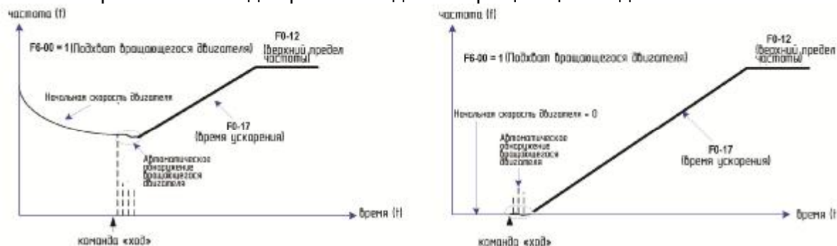
Рис. 5-10. Кривая частоты для режима подхвата вращающегося двигателя
