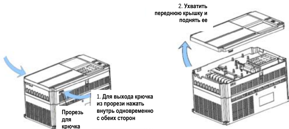
Рис. 3-13. Снятие передней крышки MD290 (металлический корпус)
