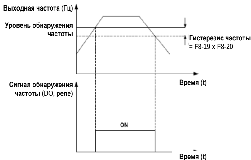
Рис. 7-23. Функция обнаружения частоты
