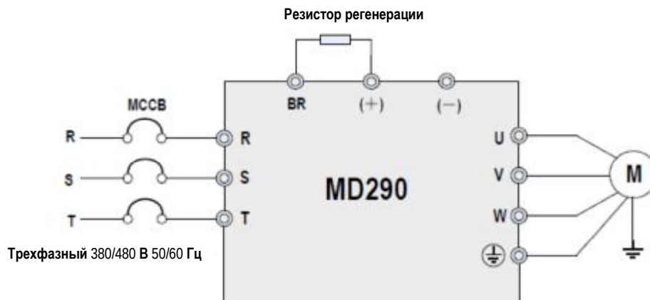
Рис. 4-2. Проводка главного контура MD290 (трехфазный ток 380 – 480 В, от 18.5G/22P до 75G/90P)
