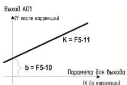
Рис. 5-32. Задание "k" и "b" выхода АО1
