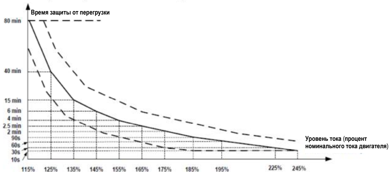
Рис. 7-31. Обратная кривая отставания по времени.
