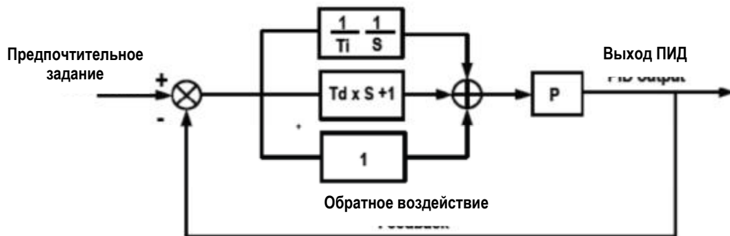
Рис. 7-33. Функция ПИД
