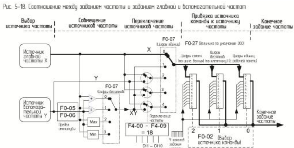
Рис. 5-18. Соотношение между заданием частоты и заданием главной и вспомогательной частот
