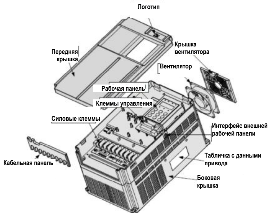
Рис. 2-3. Компоненты MD290 для металлического корпуса (трехфазный ток 380 – 480 В, от 45G/55P до 110G/132P).
