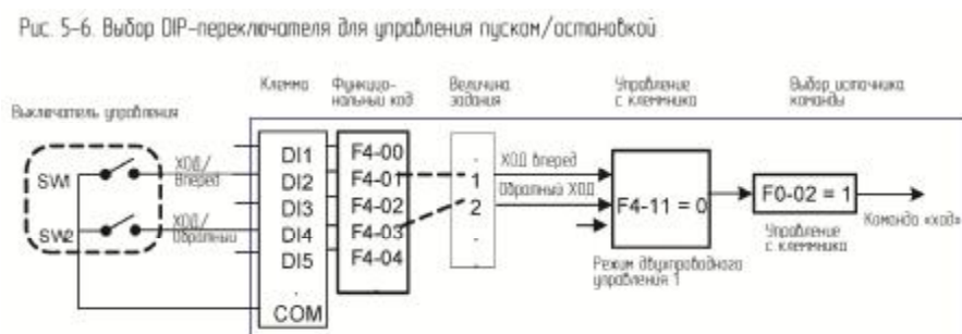
Рис. 5-6. Выбор DIP-переключателя для управления пуском/остановкой
