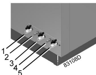
Соединительные элементы для слива и подачи воды
