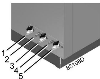
Соединения дренажа и водоснабжения
