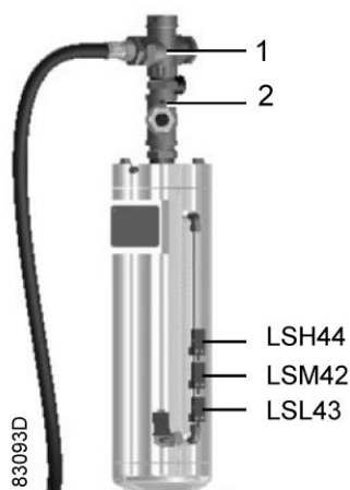
Сосуд влагоотделителя с датчиками уровня
