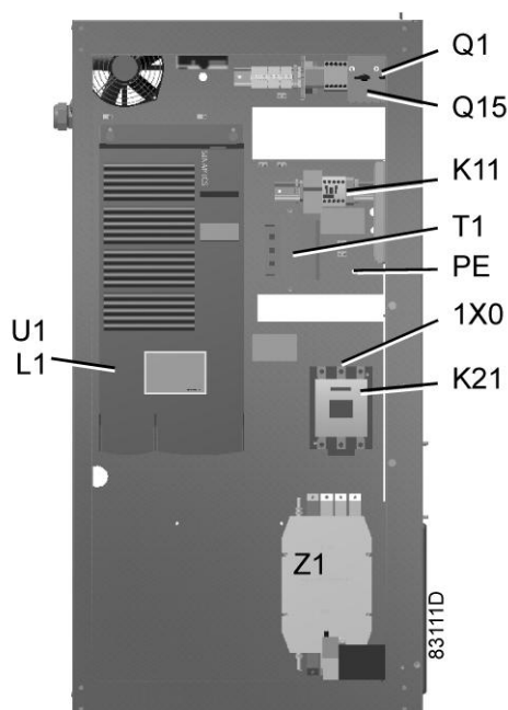
Электрический шкаф, стандартный вид
