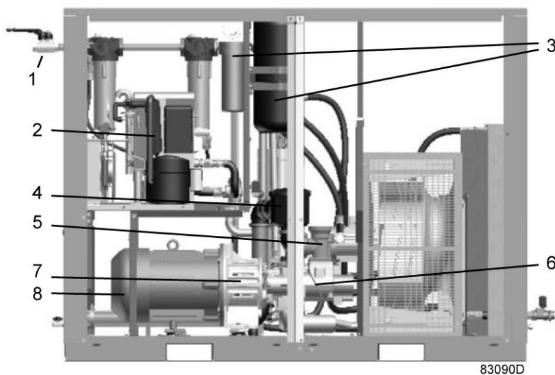
Вид сзади, компрессор с воздушным охлаждением и встроенным осушителем
