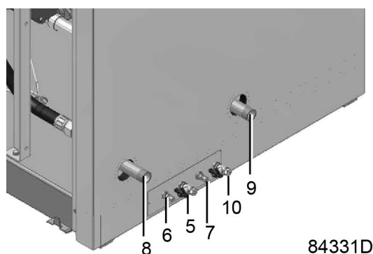
Дренаж и водоснабжение
