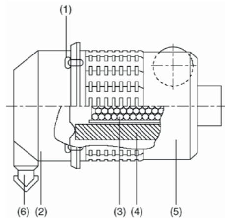
Рис. 5.2 Воздушный фильтр
