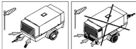
Рис. 3.2 Расположение передней части компрессора против ветра.
