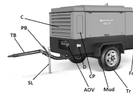
Рис. 2.1 Общий вид
