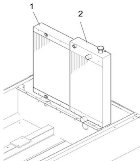
Рис. 4.2 Охладитель компрессорного масла (1) и охлаждающий моторного масла (2)
