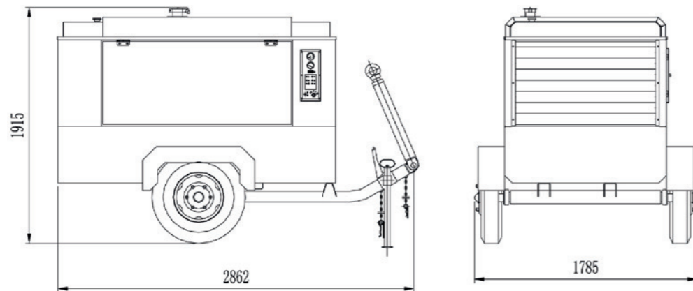
Рис. 7.1 Габаритные размеры установки
