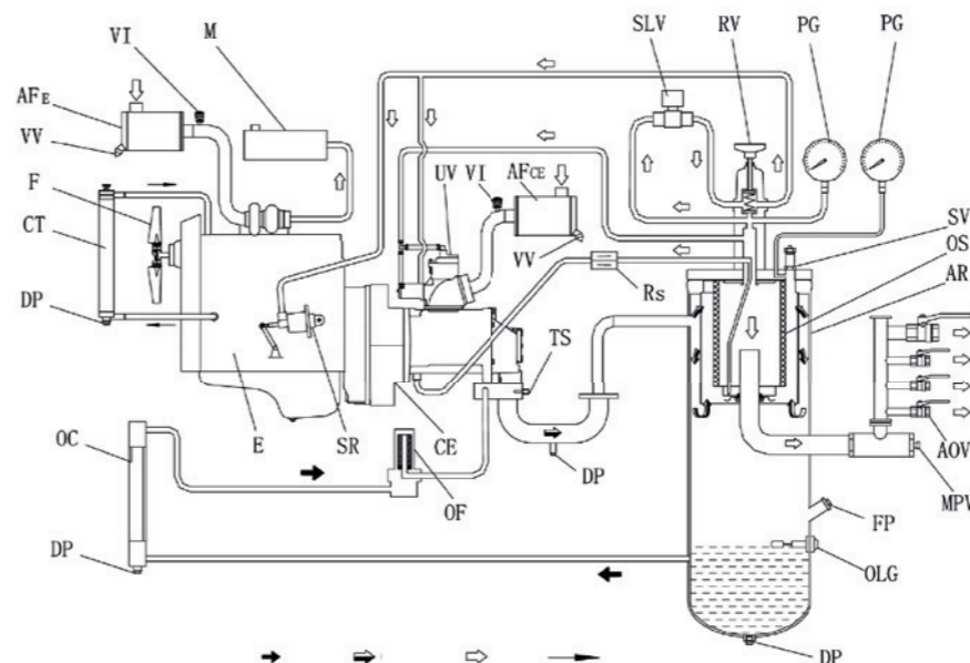
рис. 2.3 Система установки
