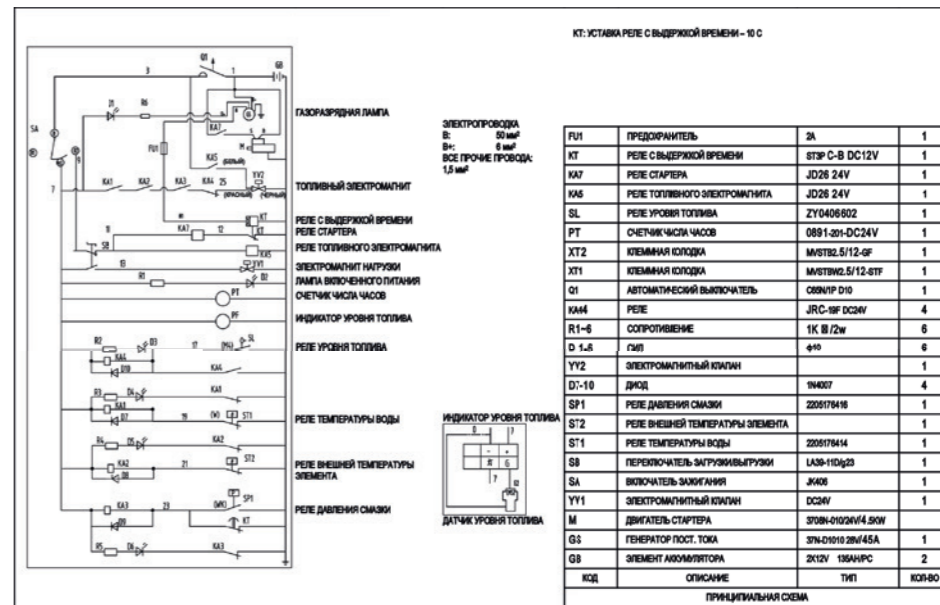
Рис. 2.4 Принципиальная схема
