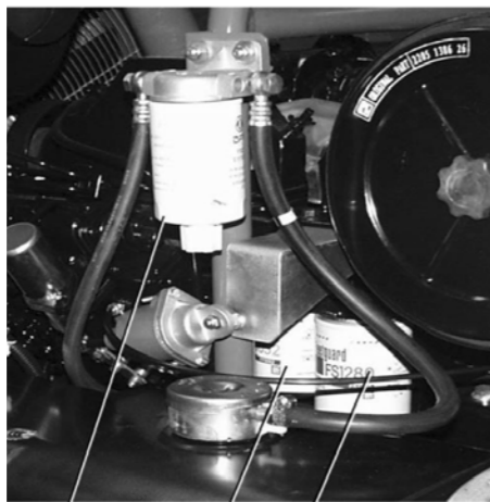
Рис. 5.4 Топливный фильтр
