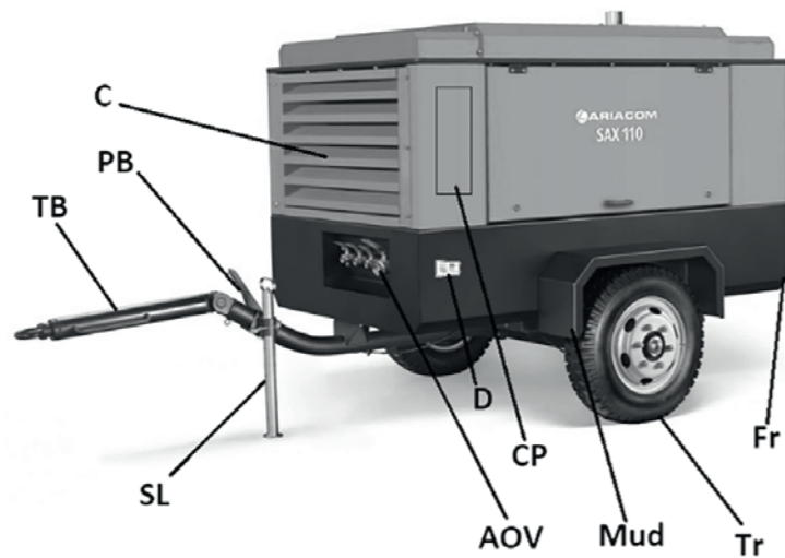
Рис. 2.2 Основные компоненты
